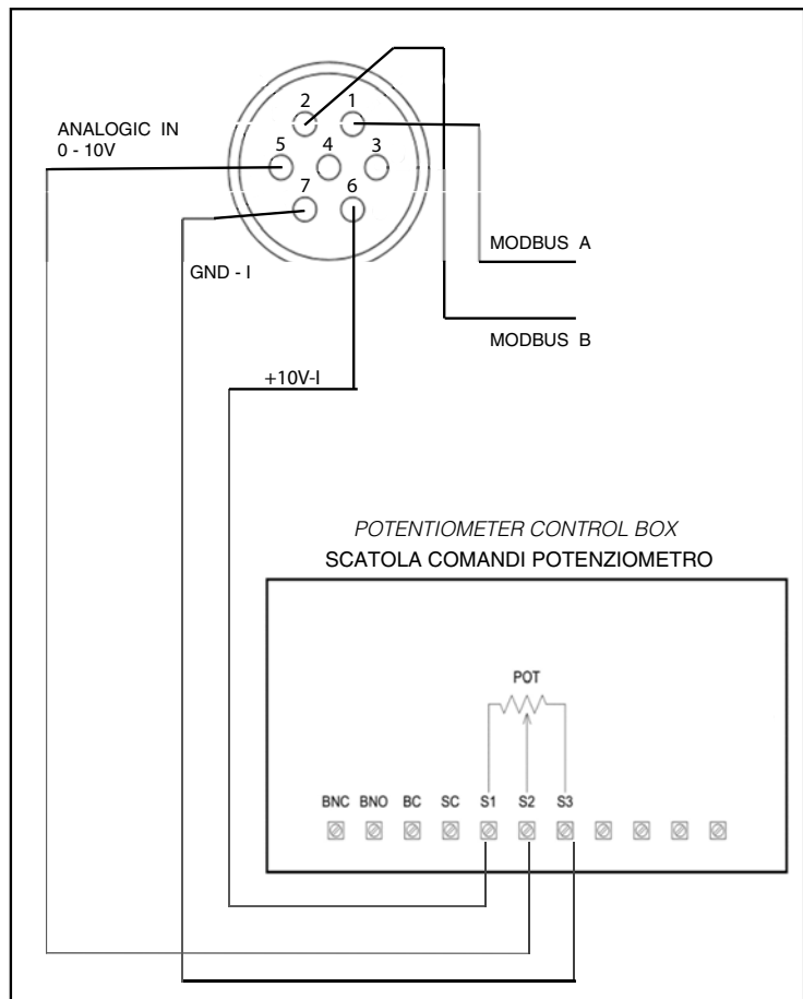
DETTAGLIO CONNESSIONI
